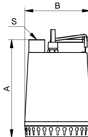
Rys. 15 Wymiary pompy
