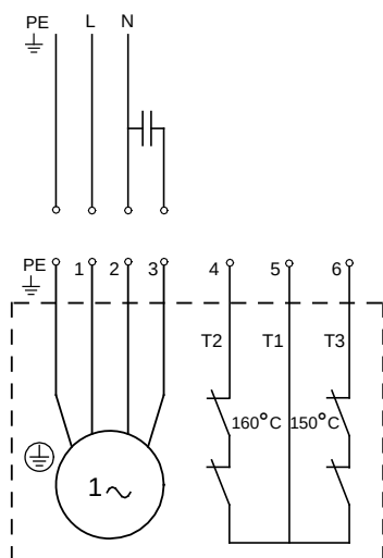
Rys. 16 Schemat połączeń dla pomp SEG jednofazowych
