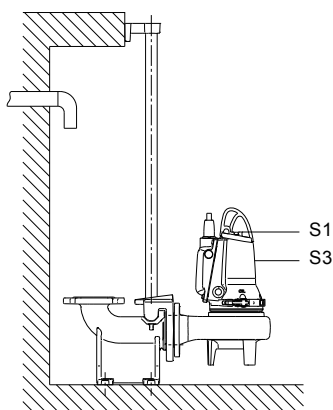
Rys. 13 Poziomy pracy
