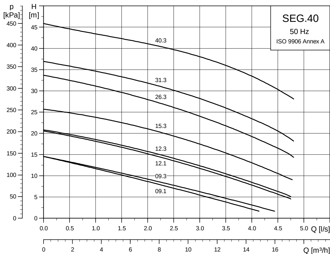
Rys. 4 Zakres pracy
