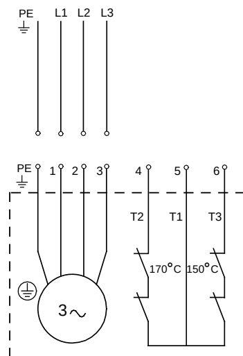
Rys. 18 Schemat połączeń dla pomp SEG trójfazowych
