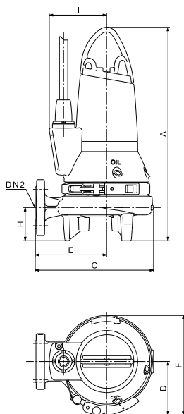
Rys. 24 Instalacja wolnostojąca
