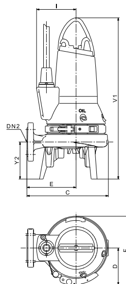
Rys. 25 Instalacja wolnostojąca z dodatkowymi nóżkami podstawy
