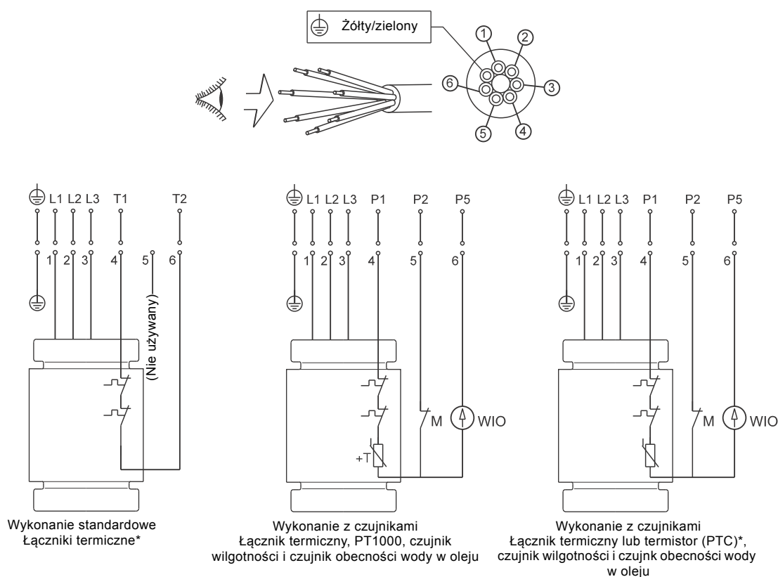
Rys. 19 Schemat połączeń, przewód 7-żyłowy, DOL
