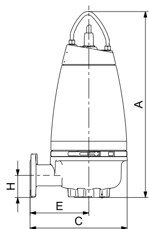
Rys. 26 Pompa SEV bez osprzętu
