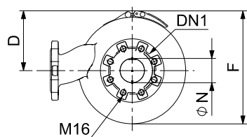
Rys. 24 Pompa SE1 bez osprzętu
