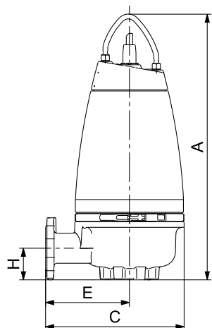
Rys. 27 Pompa SEV bez osprzętu
