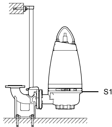
Rys. 17 Pompa zatapialna montowana na autozłączu
