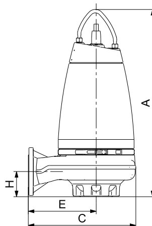
Rys. 25 Pompa SE1 bez osprzętu
