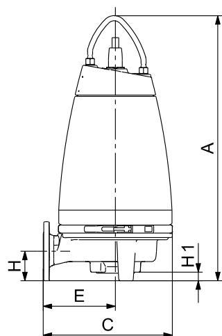
Rys. 24 Pompa SE1 bez osprzętu
