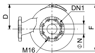
Rys. 25 Pompa SE1 bez osprzętu
