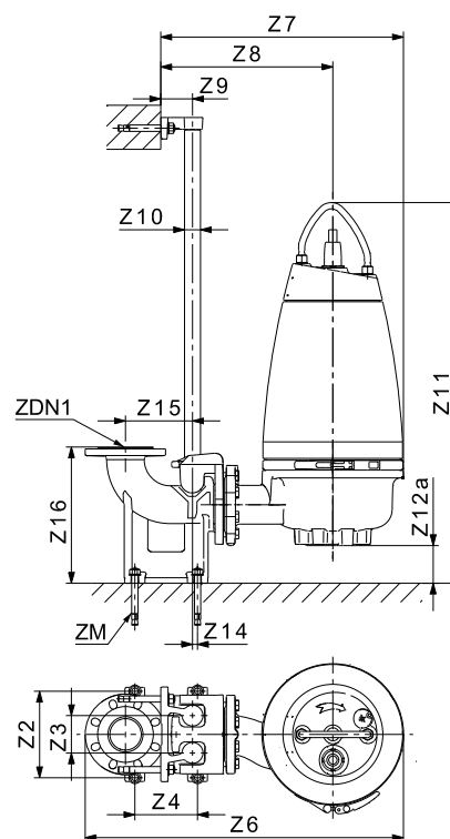
Rys. 31 SEV, pompa zatapialna na autozłączu
