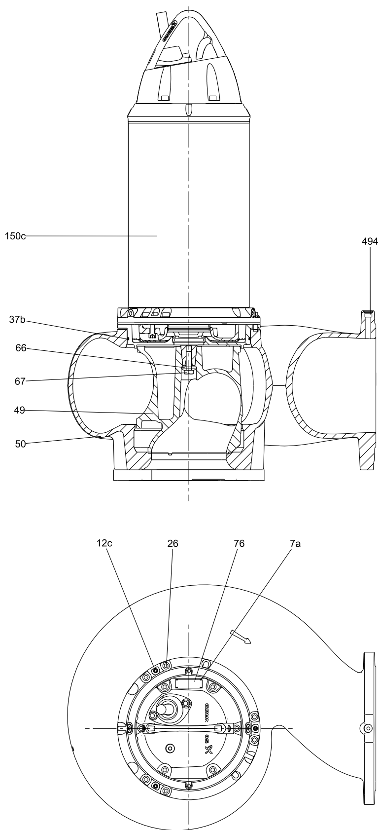
Rys. 11 Pompa SE/SL z wirnikiem tubowym S-tube
