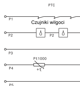
Rys. 25 czujnik GPA 1 (PTC)
