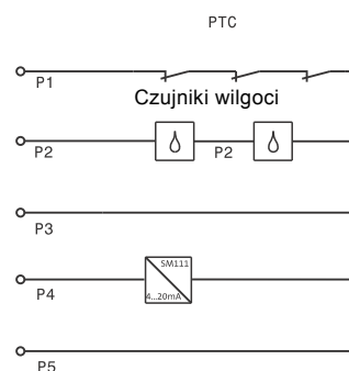
Rys. 27 czujnik GPA 2 (PTC)
