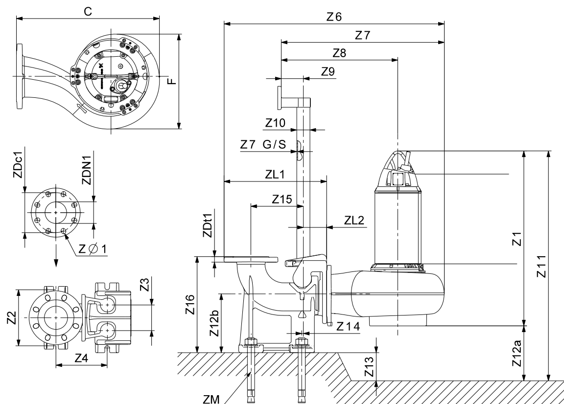
Rys. 28 Wymiary autozłaczca
