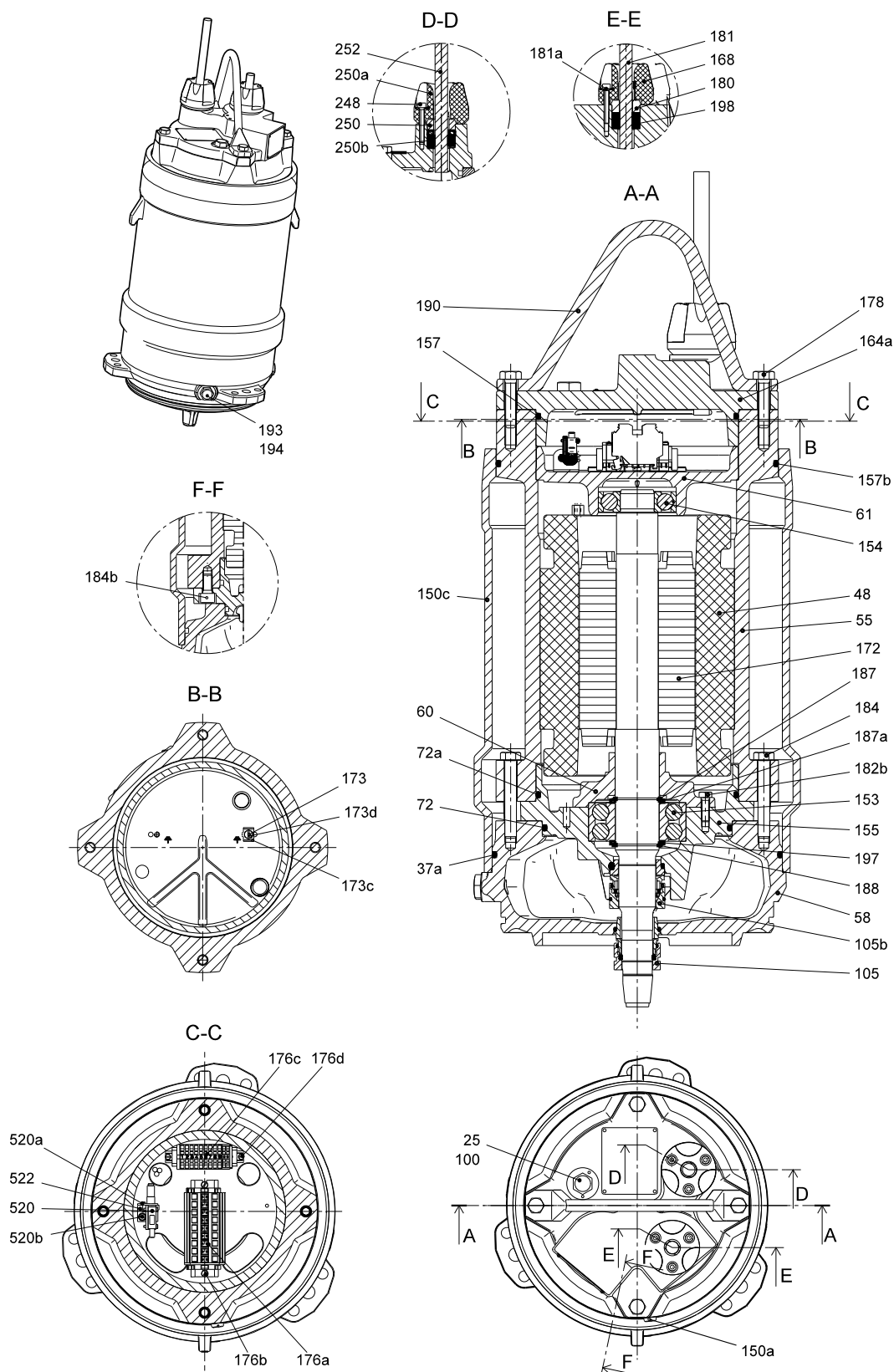
Rys. 5 Silnik w wykonaniu standardowym, bez płaszczu chłodzącego
