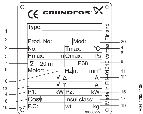
Rys. 2 Tabliczka znamionowa pompy
