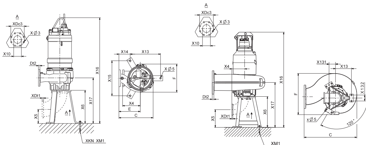
Rys. 20 Rysunki wymiarowe, montaż pionowy na sucho z podstawą
