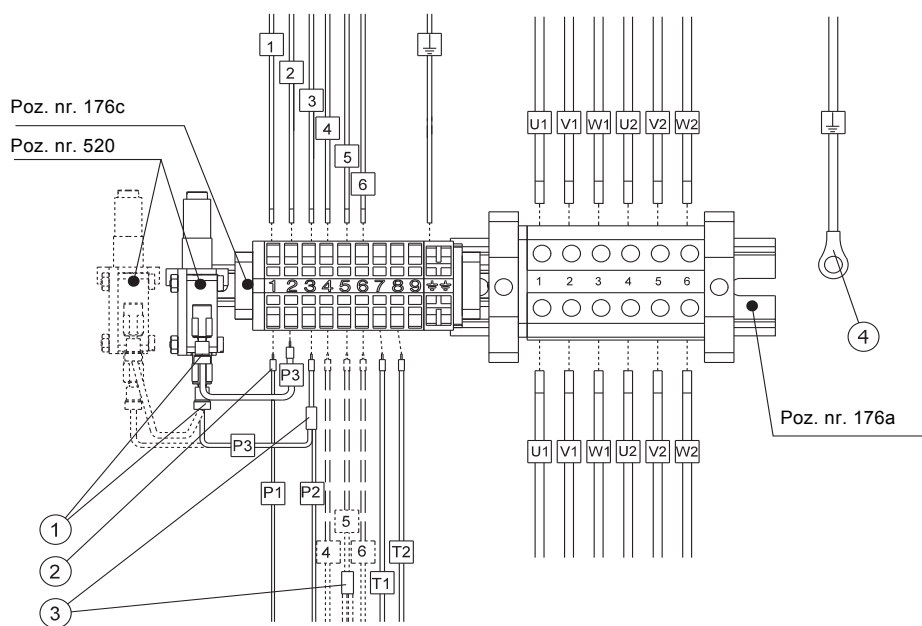
Przewody stojana
