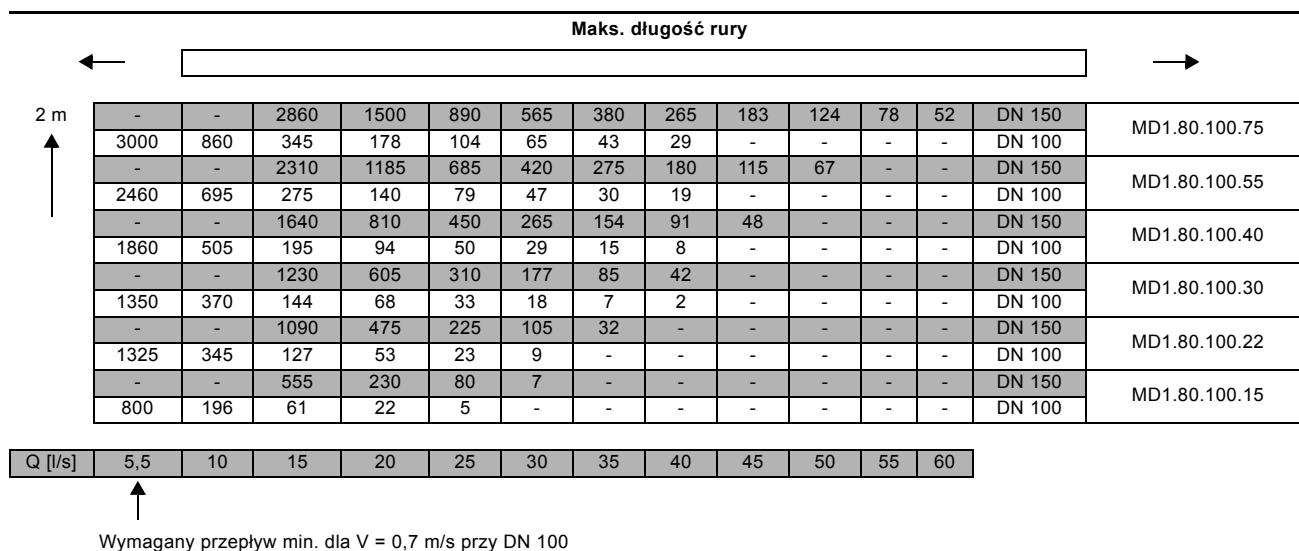
Rys. 34 Maksymalna długość rurociągów poziomych i pionowych
