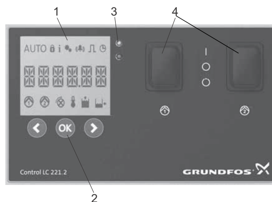
Rys. 40 Panel obsługowy sterownika do agregatów dwupompowych
