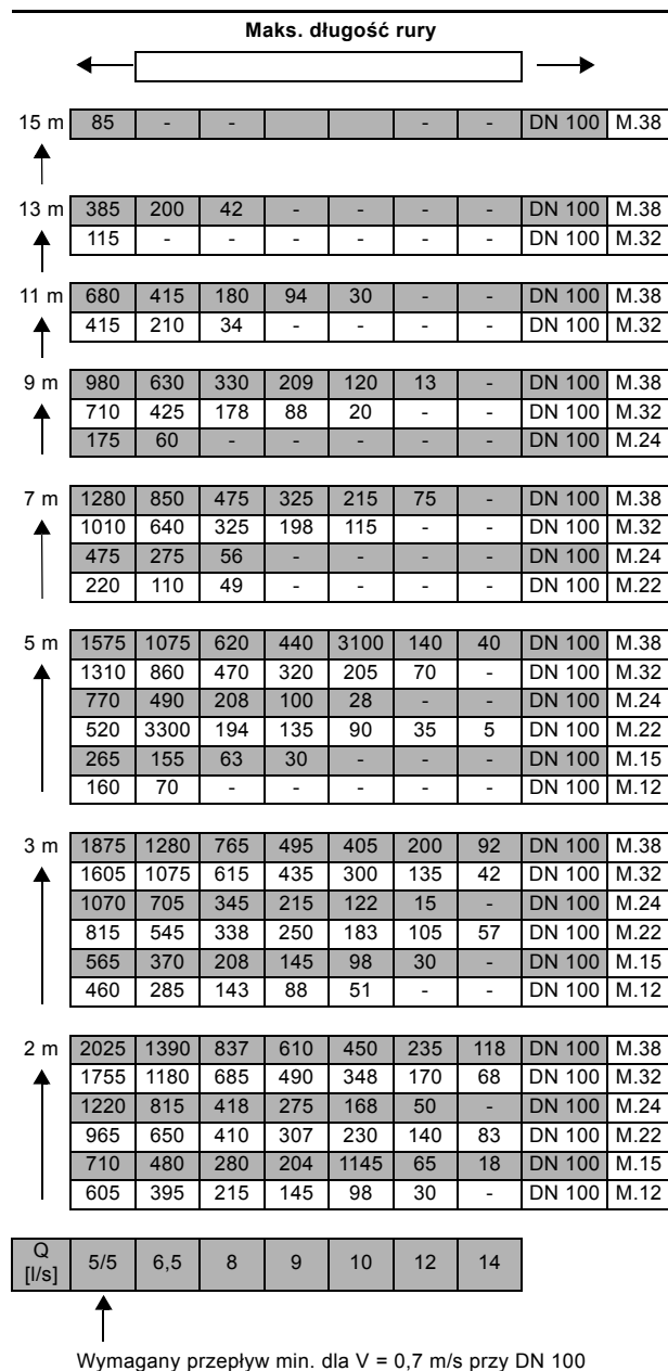
Rys. 24 Maksymalna długość rurociągów poziomych i pionowych
