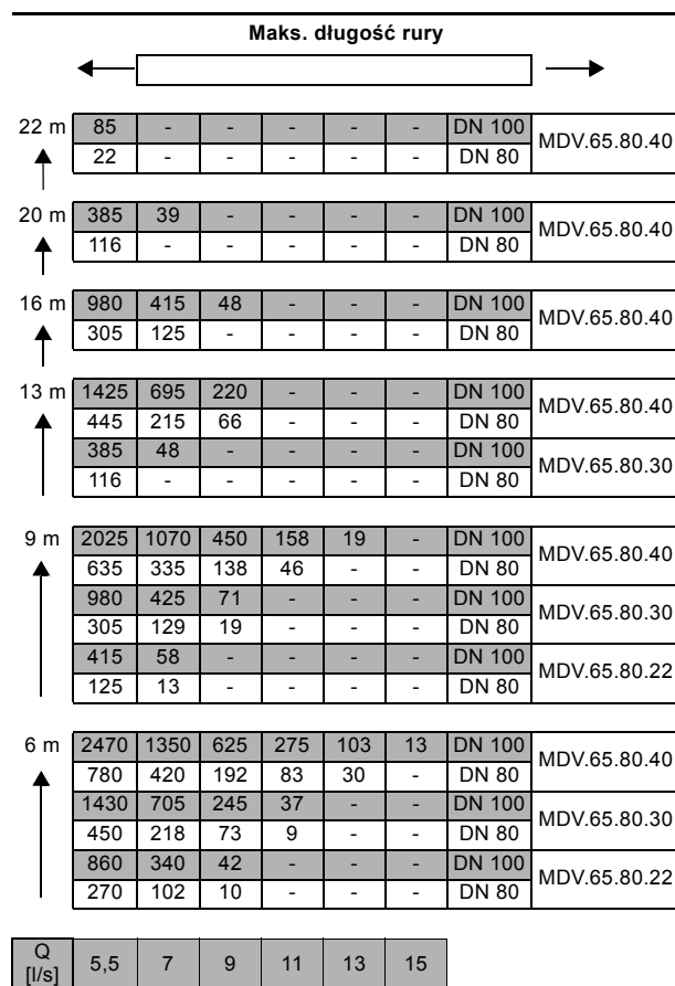
Rys. 32 Maksymalna długość rurociągów poziomych i pionowych
