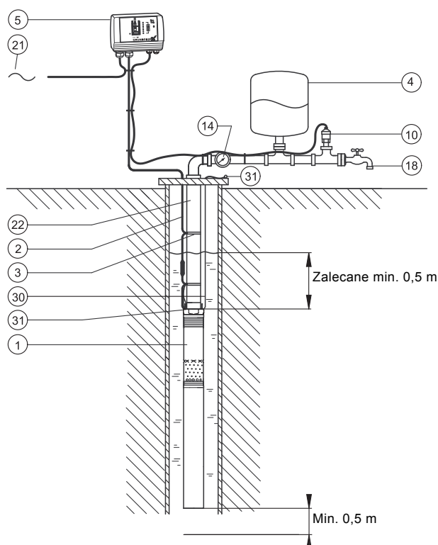
Rys. 9 Zaopatrzenie domków mieszkalnych w wodę z CU 301
