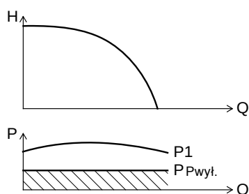
Rys. 2 Zabezpieczenie przed suchobiegiem
