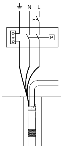
Rys. 30 Schemat połączeń do sieci zasilającej
