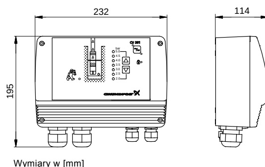
Rys. 19 Rysunek wymiarowy CU 301
