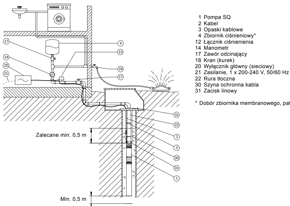
Rys. 7 Domowe instalacje zasilania w wodę
