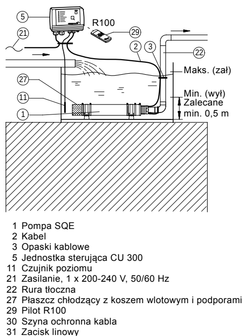
Rys. 12 Opróżnianie lub napełnianie zbiornika
