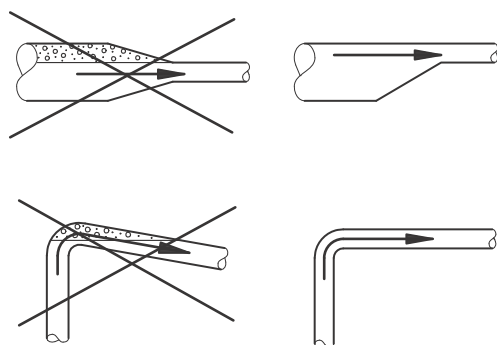
Rys. 2 Zalecenia rurociągów
