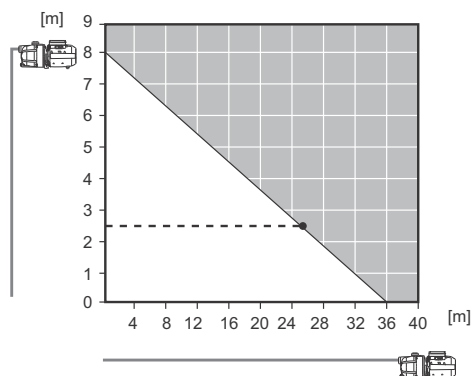
Rys. 1 Zalecana maksymalna wysokość ssania lub maksymalna długość przewodu ssawnego
