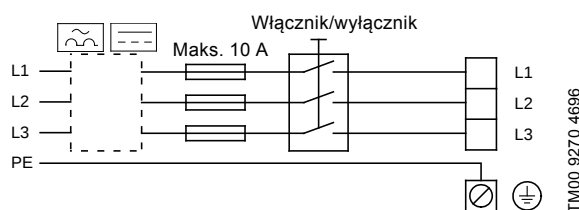
Rys. 5 Schemat połączeń - wersja 3-fazowa, 2,2 - 7,5 kW
