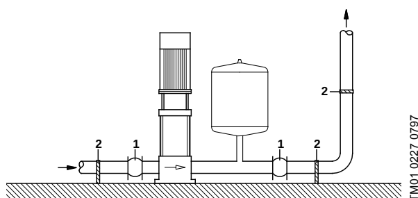
Rys. 3 Montaż mechaniczny
