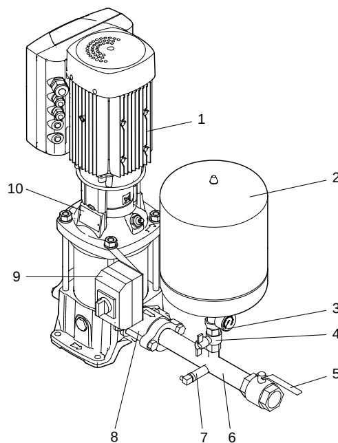
Rys. 2 Budowa Hydro Solo-E
