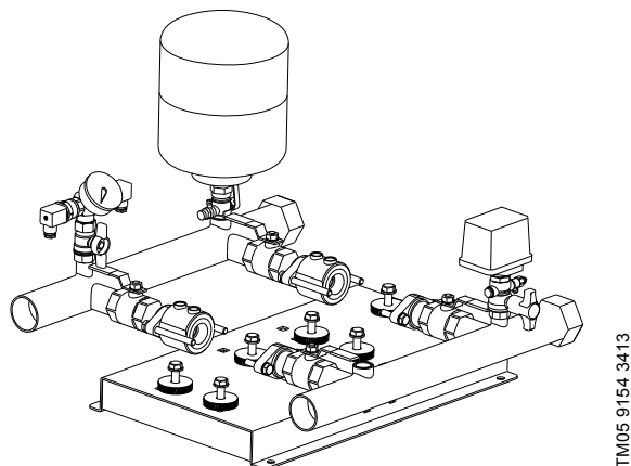
Rys. 6 Rama podstawy, kolektory i zawory
