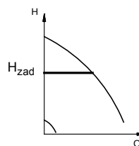
Rys. 14 Tryb regulacji stałego ciśnienia
