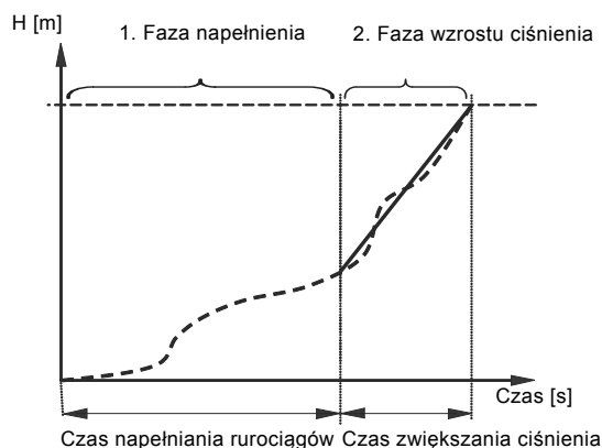
Rys. 16 Faza napełniania i podnoszenia ciśnienia
