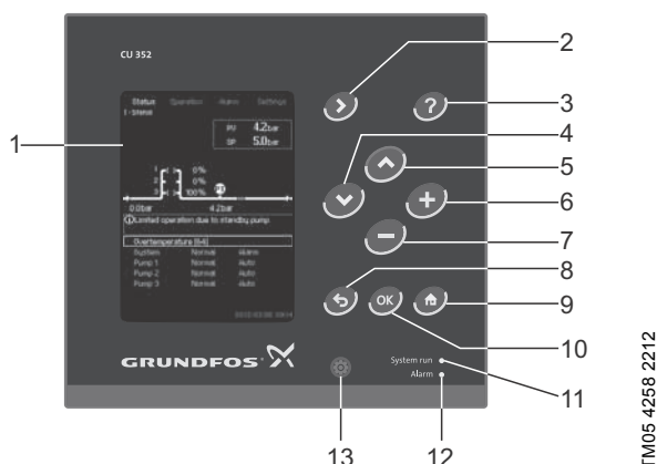
Rys. 9 Panel sterowania CU 352
