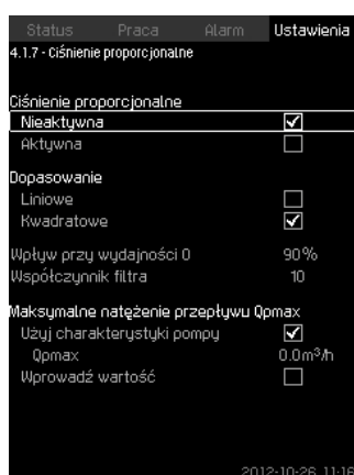
Rys. 26 Ciężnienie proporcjonalne
