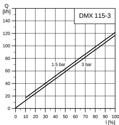
DMX 115-3
