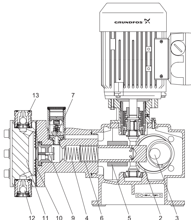
Rys. 14 Rysunek przekrojowy,
