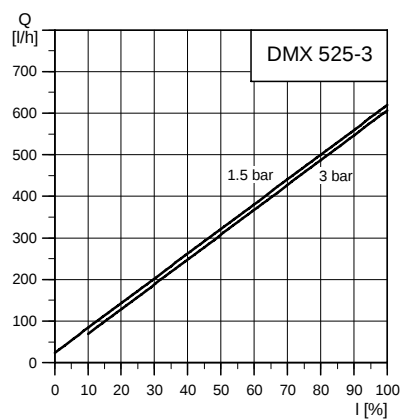
DMX 525-3
