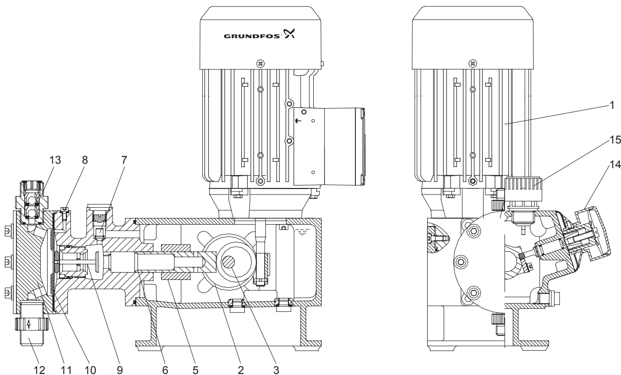
Rys. 12 Rysunek przekrojowy,
