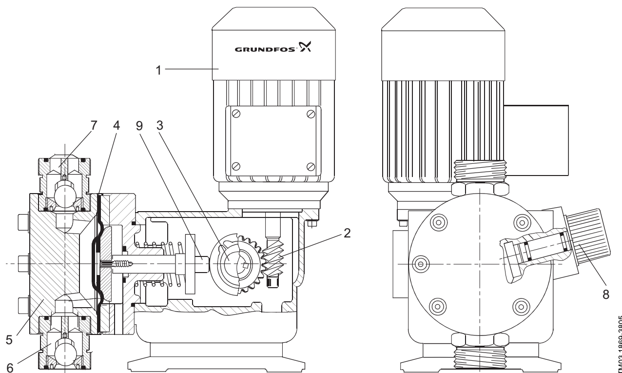
Rys. 10 Rysunek przekrojowy,
