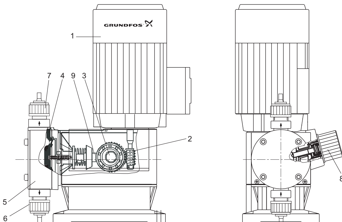
Rys. 9 Rysunek przekrojowy,
