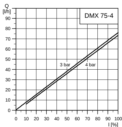
DMX 75-4
