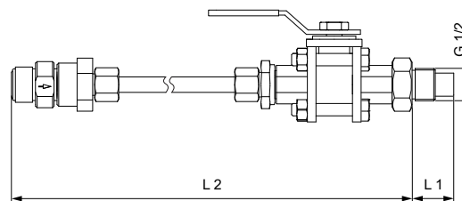
Rys. 39 Zawór dozujący do cieczy gorących z zaworem kulowym
