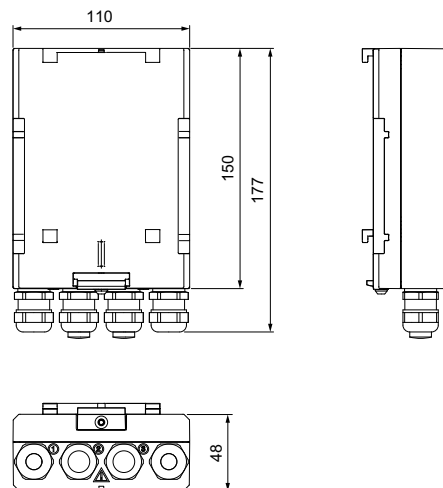
Rys. 28 E-box, wymiary
