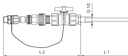
Rys. 38 Zawór dozujący, wyjmowalny do czyszczenia
