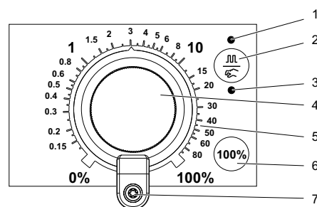
Rys. 8 Elementy robocze DDE
