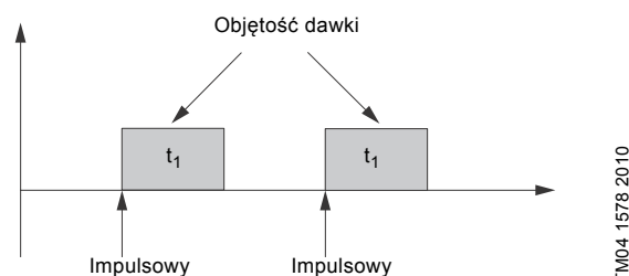
Rys. 12 Impulsowe sterowanie dawką
