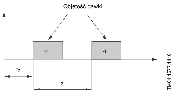
Rys. 13 Cykliczny przełącznik dozowania
