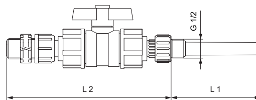
Rys. 37 Zawór dozujący z zaworem kulowym
