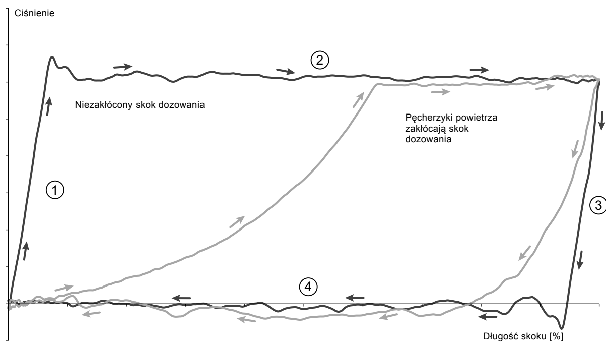
Rys. 18 Wykres indykatorowy
