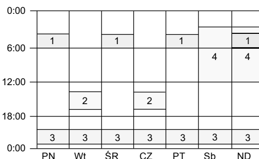
Rys. 14 Tygodniowy przełącznik czasowy (przykład z 4 procedurami)
