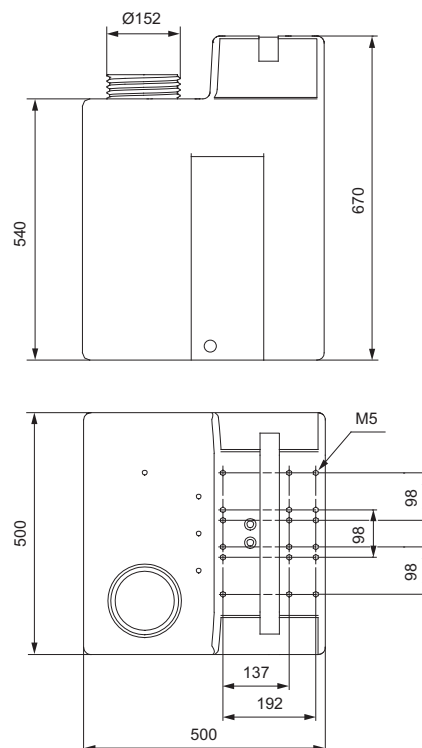
Rys. 47 Zbiornik kwadratowy, wymiary
