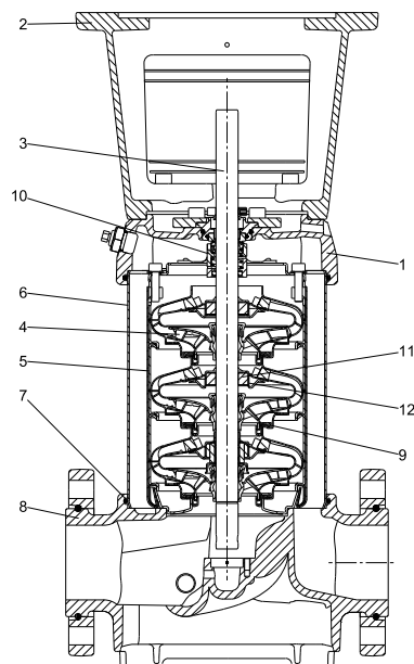
Rysunek przekrojowy
