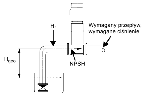
Rys. 11 Dane doboru
