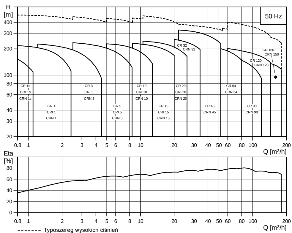
Rys. 2 Zakres stosowalności CR, CRI i CRN
