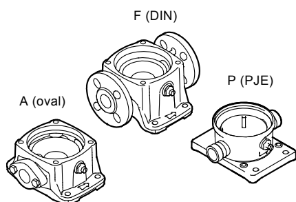
Rys. 13 Przylączy pompy
