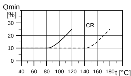
Rys. 17 Wydajność minimalna
