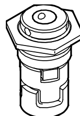
Rys. 14 Uszczelnienie wału (kasetowe)
