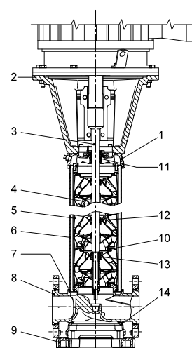
Rysunek przekrojowy
