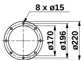
Pompa z kołnierzem Grundfos
