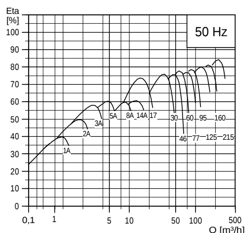
Rys. 1 Sprawność pompy/silnika w odniesieniu do przepływu
