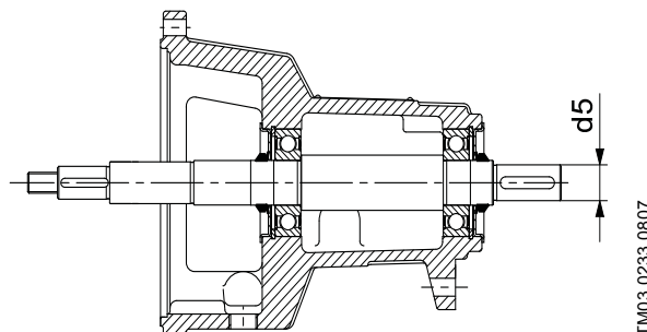
Rys. 15 Korpus łożyskowy i wał
