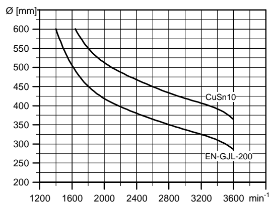
Rys. 49 Dopuszczalna maksymalna prędkość obrotowa
